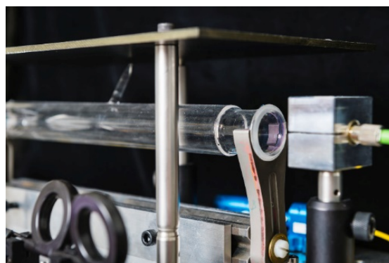
Figure 1: cellule d'acétylène
